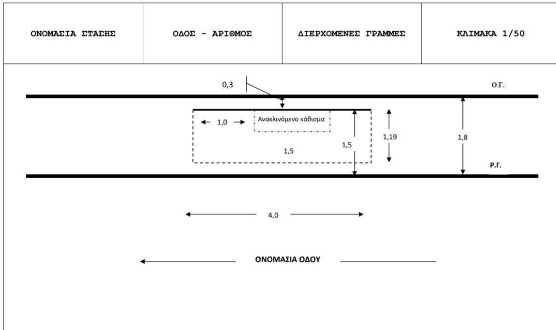
Ενδεικτικό σκαρίφημα τοποθέτησης στεγάστρου τύπου Β
