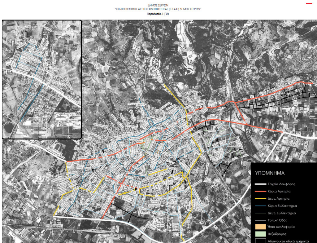
Σχήμα 4-2: Λειτουργική ιεράρχηση οδικού δικτύου
