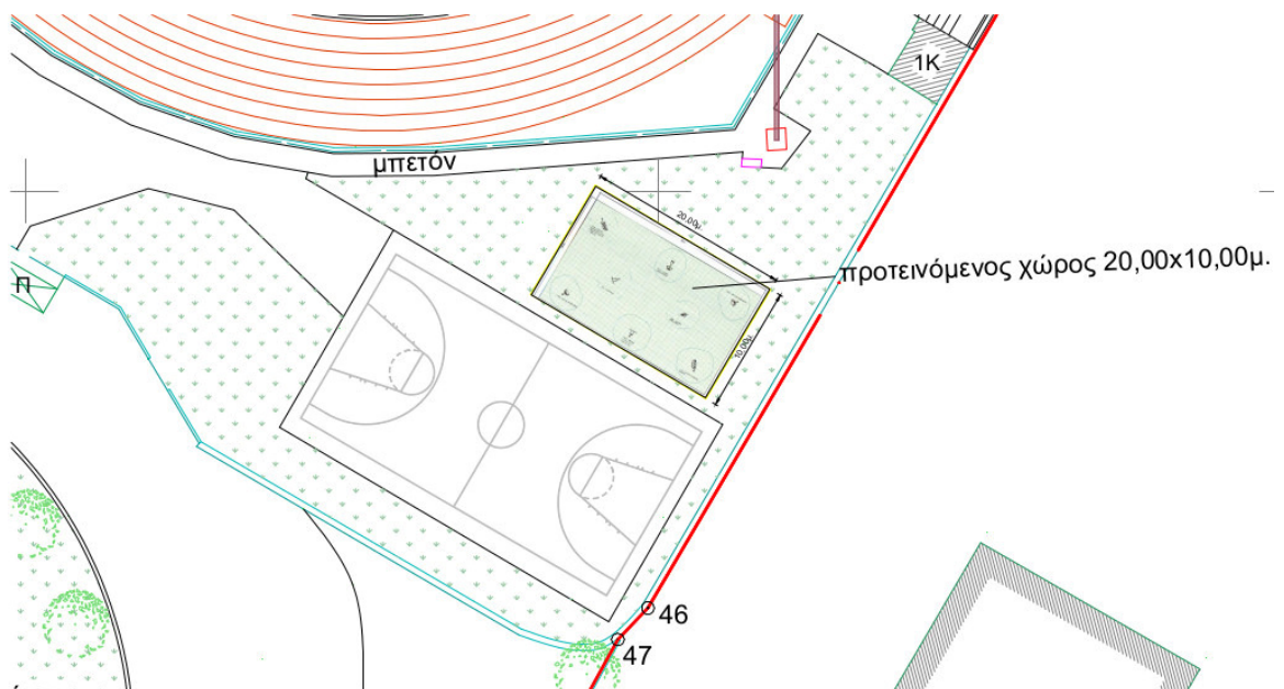
Εικόνα 4 : Χωροθέτηση εντός του ακινήτου, της εγκατάστασης οργάνων γυμναστικής εμβαδού περίπου 200τ.μ. (20x10μ.).
