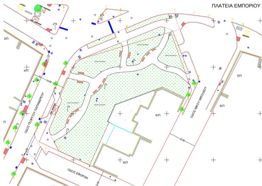
Εικόνα 3 : Προτεινόμενος χώρος εγκατάστασης οργάνων γυμναστικής (απόσπασμα σχεδίου).
